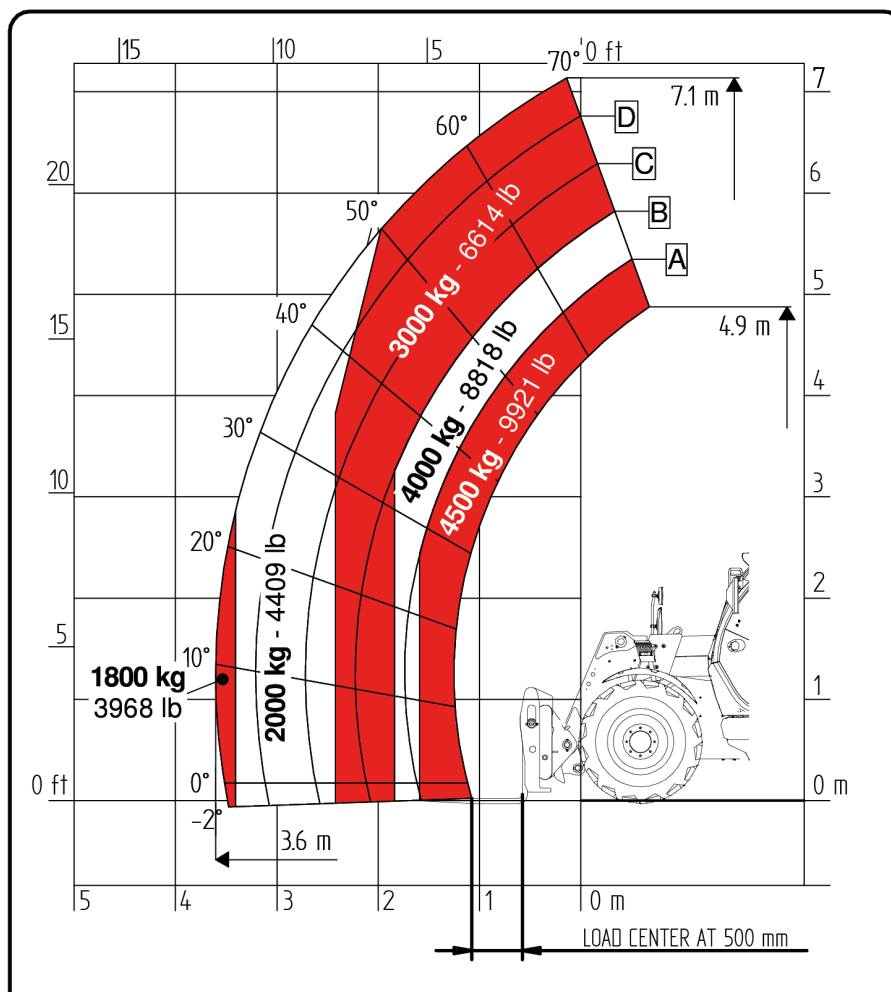
Alapkivitel · Gyári terhelési diagram
